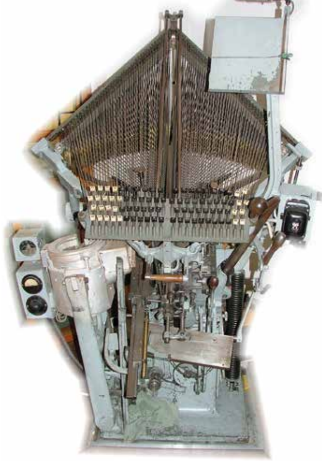
EINE »TYPOGRAPH«-SETZMASCHINE
